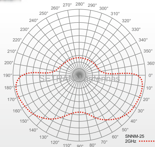
E-PLANE
